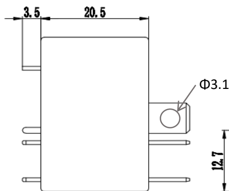
外形尺寸图
