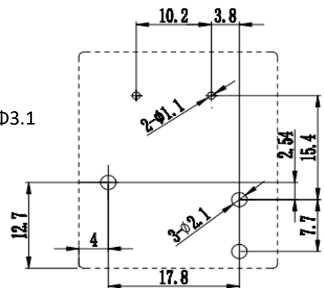
安装尺寸图
