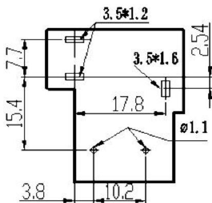
安装尺寸图
