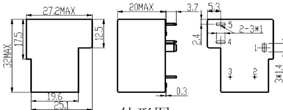
外形图
