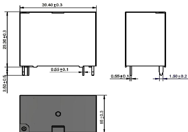
外形图
