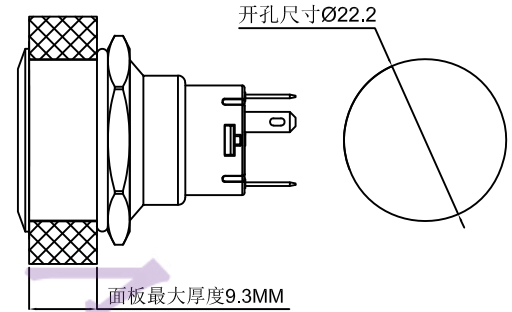
安装视图
