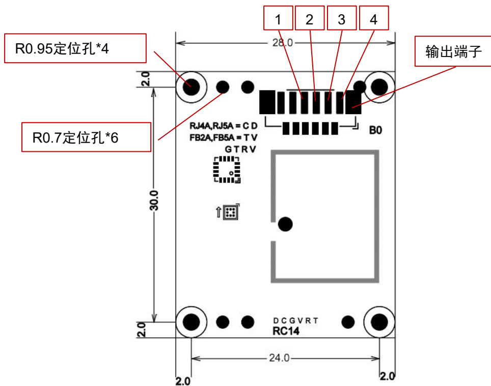
正面视图(屏蔽盖朝上)
