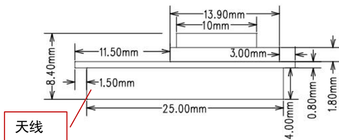
侧面视图
