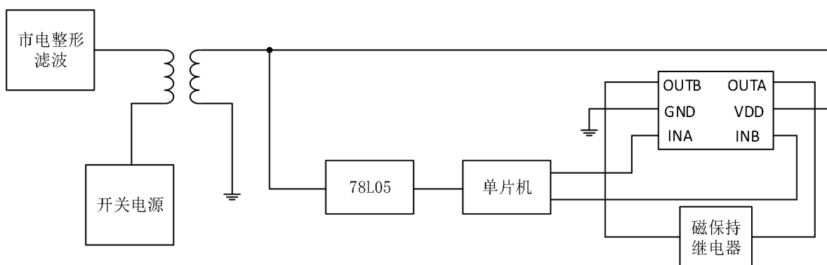
图5 应用电路示意图
