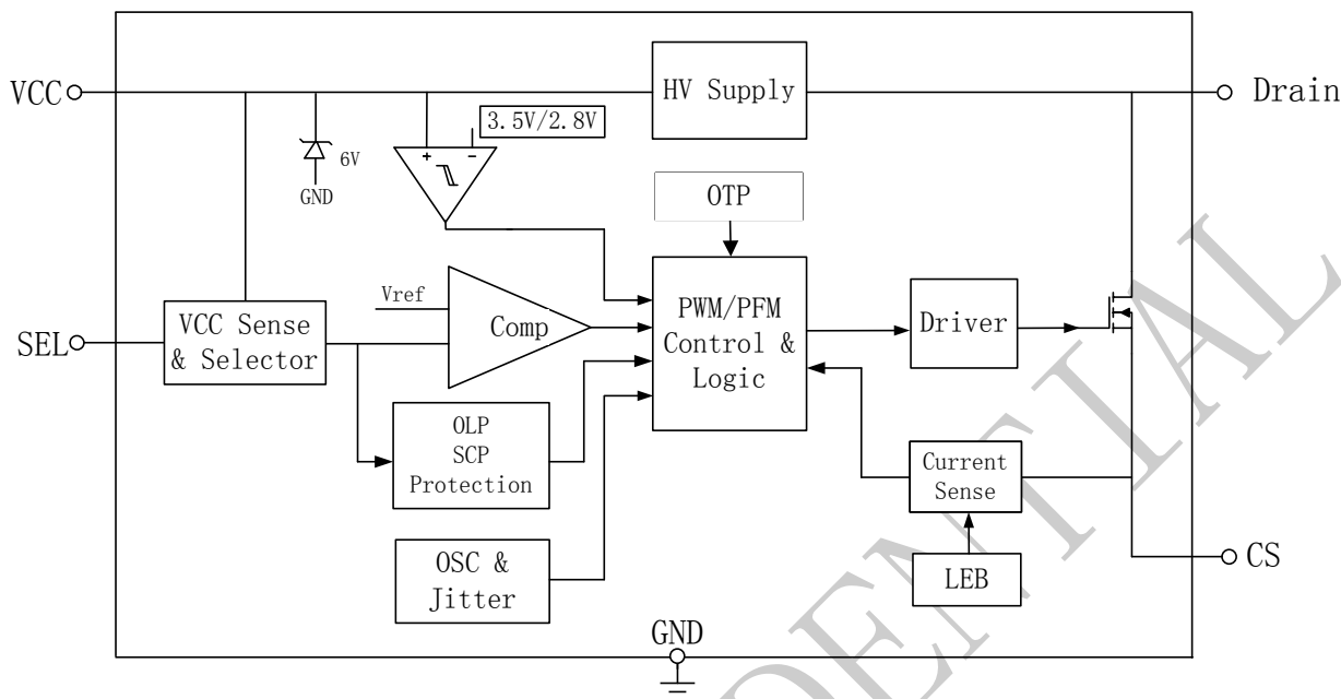
图 4 BP2525X 内部框图
