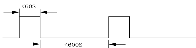
图 3 瞬时脉冲示意图
