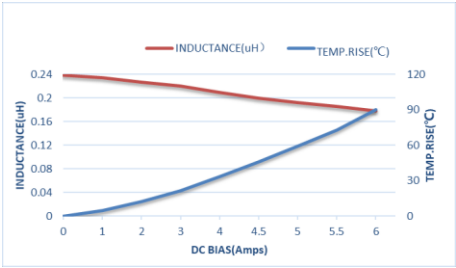
ZET-CORE-160808STR22MBCA
