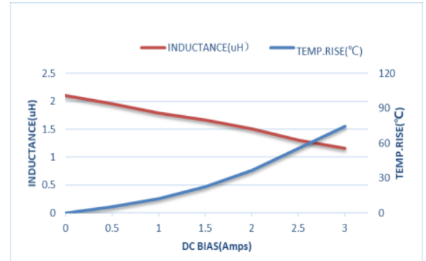
ZEMS201265-2R2M
