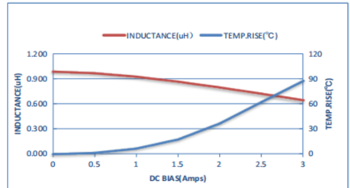
ZETC160865S1R0MGT-LF
