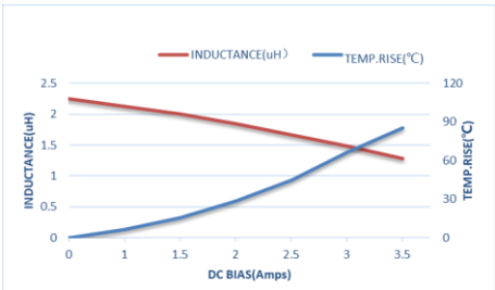
ZETC201608S-2R2MT-LF
