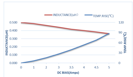
ZEPIM201208S-R47M
