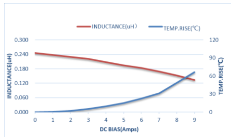
ZEPIM201208S-R24M
