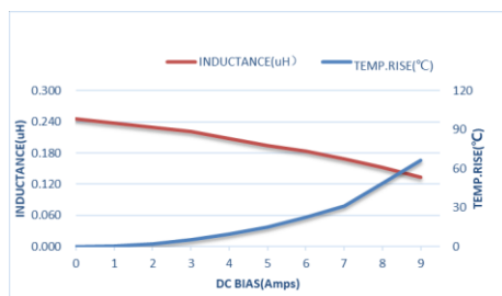
ZETC201208SR24MBT-LF
