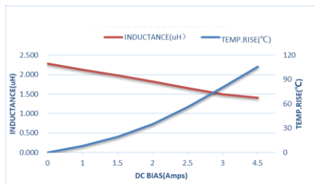
ZETC201208S2R2MBT-LF
