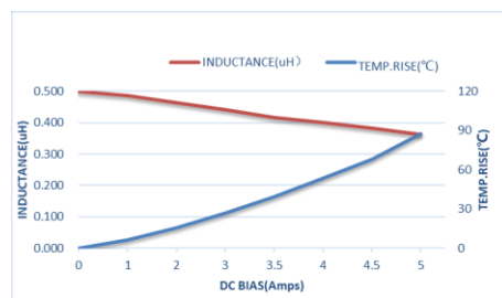
ZETC201208SR47MBT-LF
