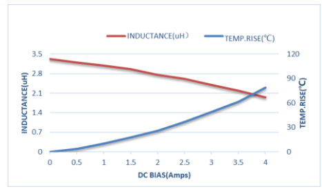
ZETC252012S3R3MBT-LF
