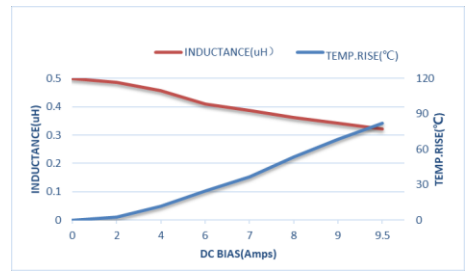
ZETC252012SR47MBT-LF
