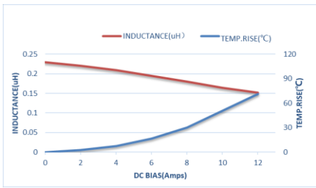
ZETC252012SR24MBT-LF
