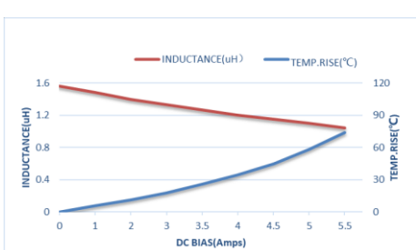
ZETC252012S1R5MBT-LF
