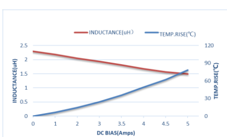
ZETC252012S2R2MBT-LF
