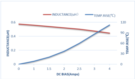
ZETC160808SR56MBT-LF
