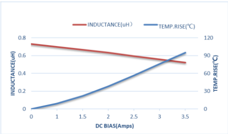
ZETC160808SR68MBT-LF
