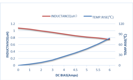
ZETC252012S1R0MBT-LF
