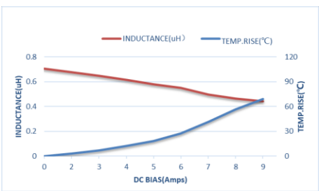
ZETC252012SR68MBT-LF
