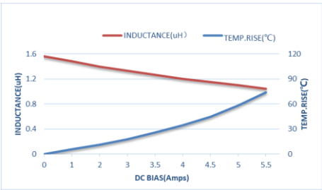
ZETC252012S1R5MBT-LF
