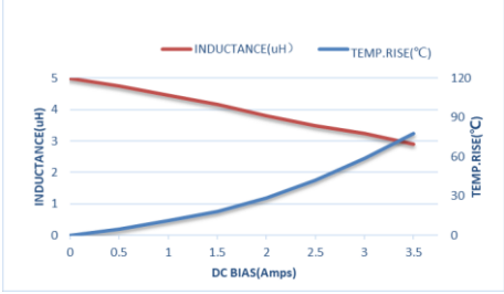
ZETC252010S4R7MBT-LF
