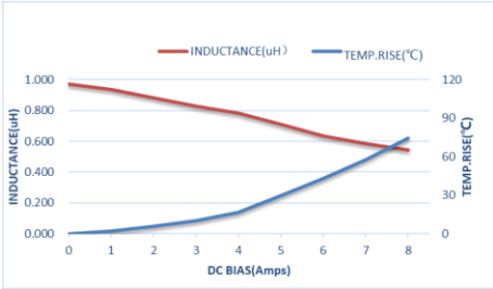
ZETC252010S1R0MBT-LF
