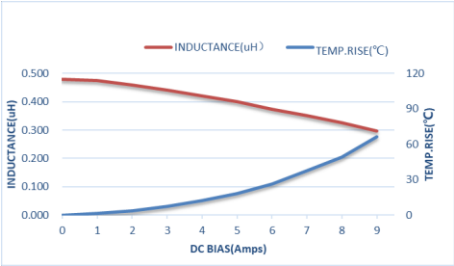
ZETC252010SR47MBT-LF
