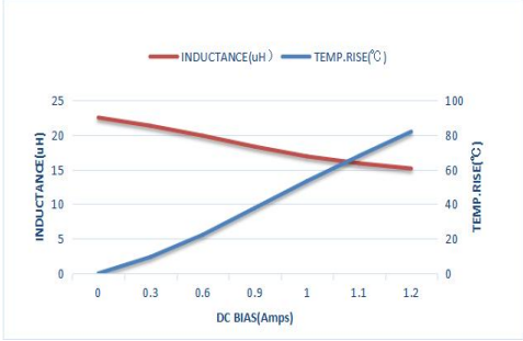
ZETC252010S220MBT-LF
