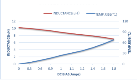
ZETC252010S100MBT-LF
