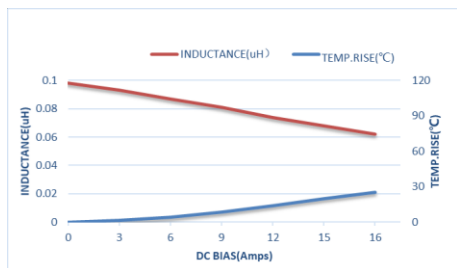
ZETC201612S-R10MT-LF
