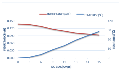
ZETC201612S-R15MT-LF
