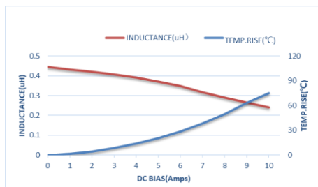
ZETC201612S-R47MT-LF
