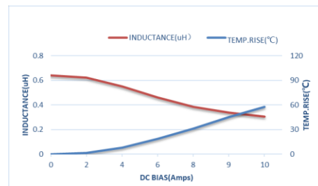
ZETC201612S-R68MT-LF
