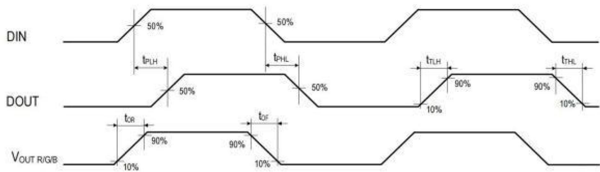
Fig. HWS2811-TD动态参数测试示意图
