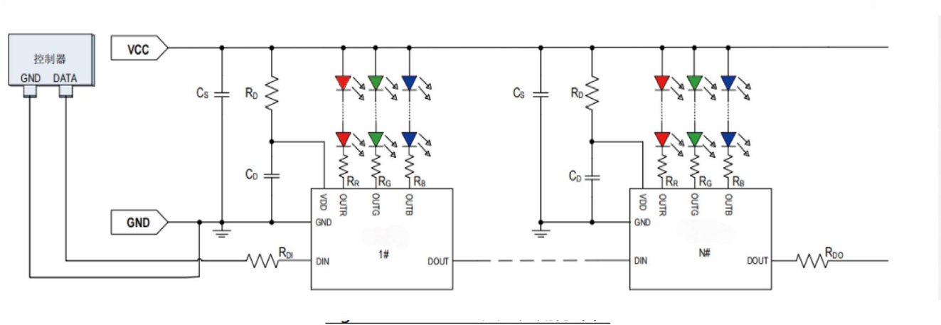
Fig. HWS2811-TD典型应用方案图
