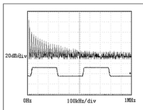
图 11:传输 20kHz 信号时 TD308X 系列驱动输出波形和 FFT 图
