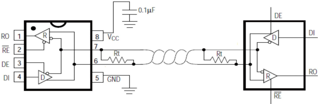
图 1: TD308X系列 典型半双工应用电路
