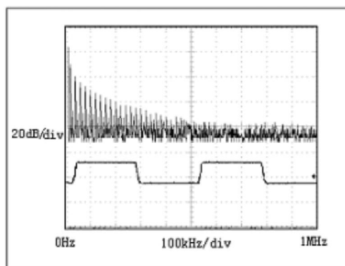
图 11:传输 20kHz 信号时 TD308X 系列驱动器输出波形和 FFT 图
