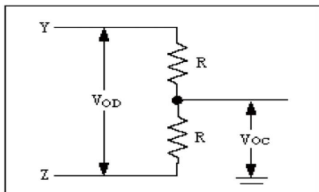
图 2:驱动器 DC 测试负载
