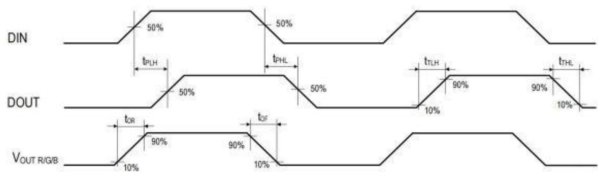
Fig. HTM1903-TD动态参数测试示意图
