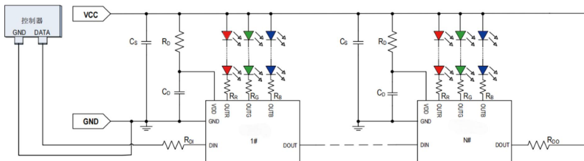
Fig. HTM1903-TD典型应用方案图
