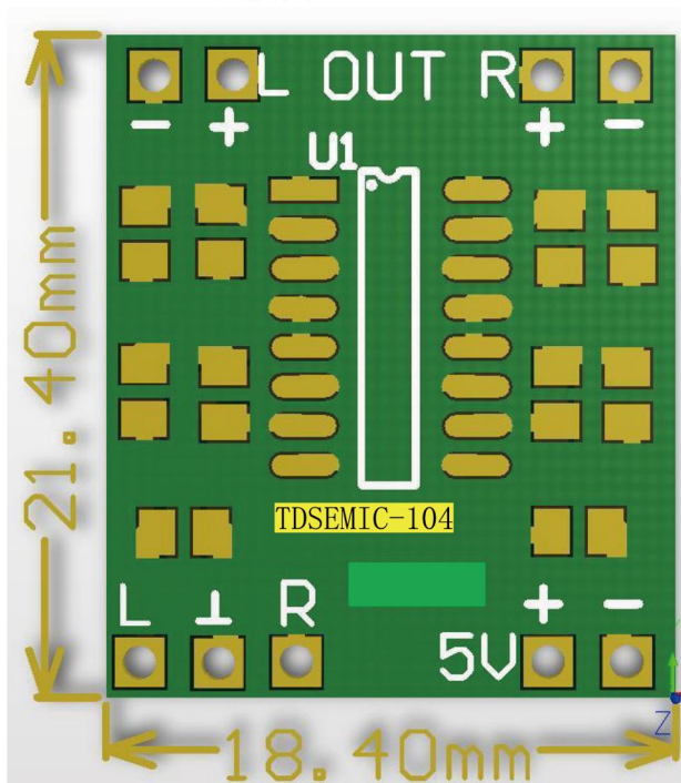
PCB 正面图:
