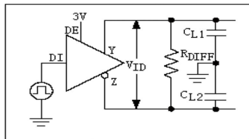
图 4: 驱动器定时测试负载
