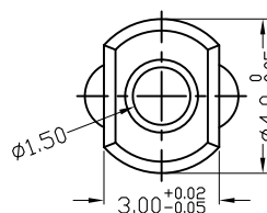
轴心部尺寸详图
