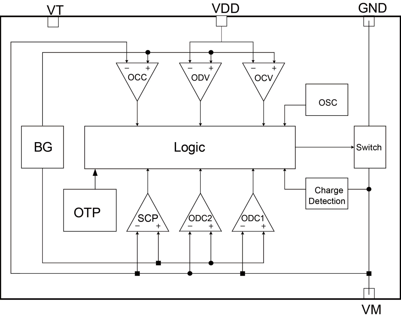
功能框图
