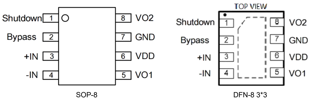
图 1. SSM2211 的管脚定义图
