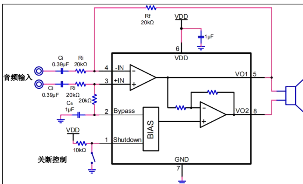
图 3. SSM2211 差分输入模式电路图
