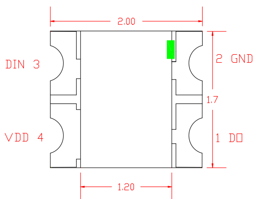
正面图
