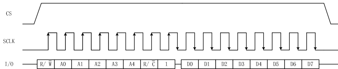
图 5.2 读数据
