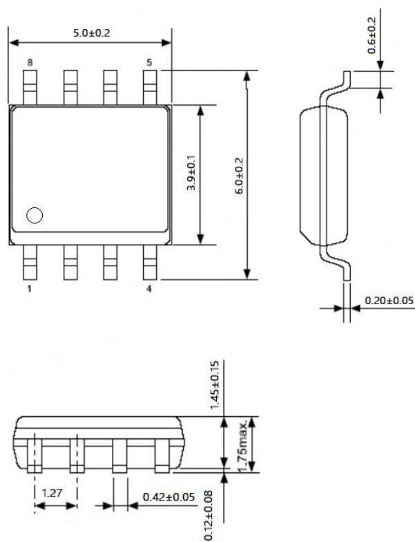
SD8908 SOP8 150mil 封装及盘装尺寸图
