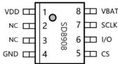
图 3.1 管脚定义
