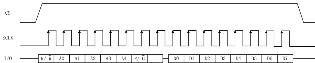
图 5.3 写数据
