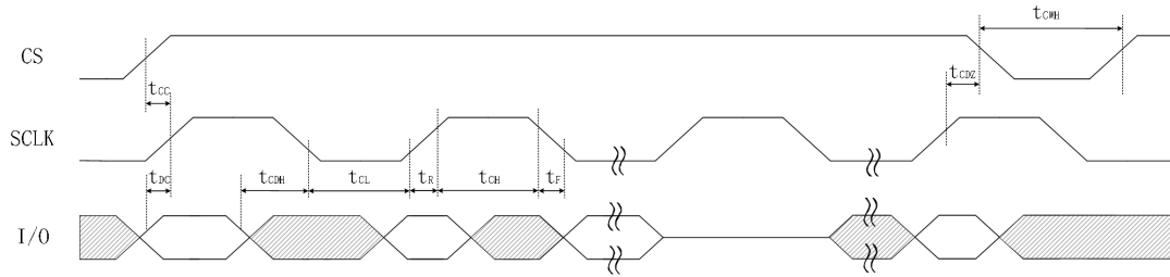
图 5.7 写数据波形图
