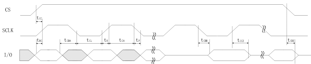
图 5.6 读数据波形图
