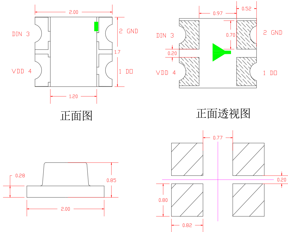
建议焊盘尺寸
