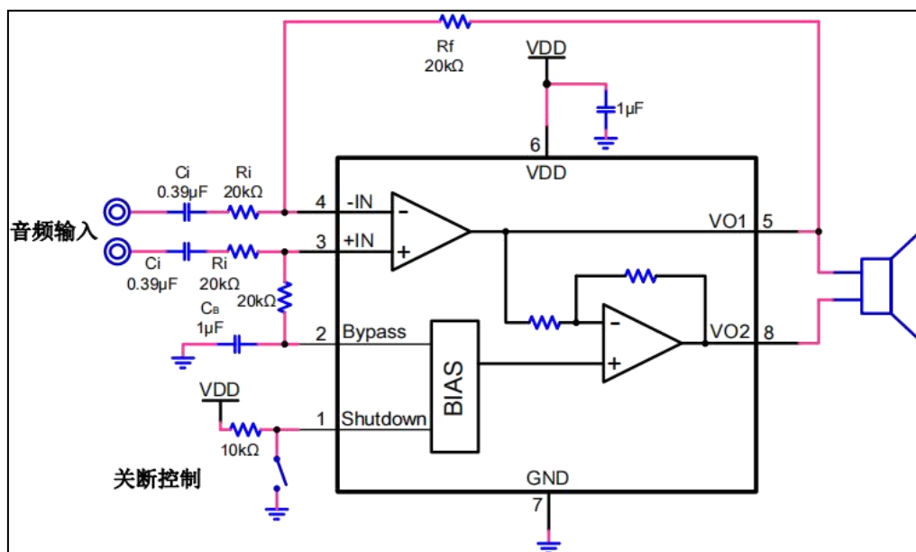
图 3. TPA4861 差分输入模式电路图
