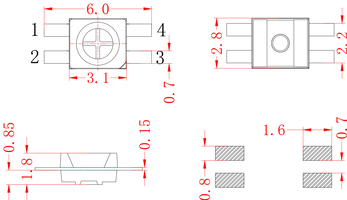
建议焊盘尺寸
