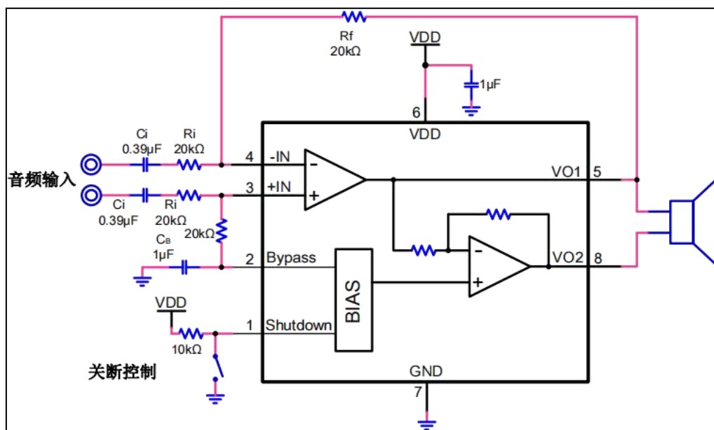
图 3. LM4876 差分输入模式电路图
