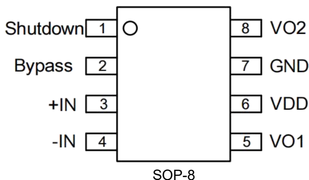
图 1. LM4876 的管脚定义图
