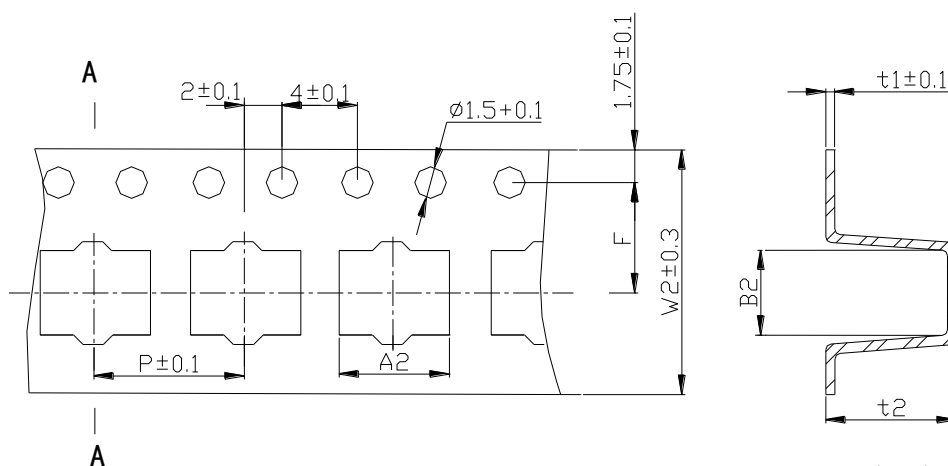
A-A断面
