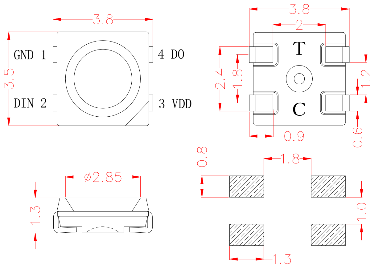
建议焊盘尺寸
