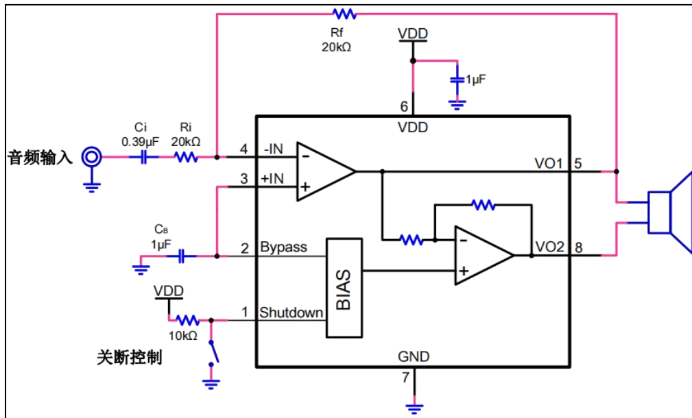
图 2. TS4871 单端输入模式电路图
