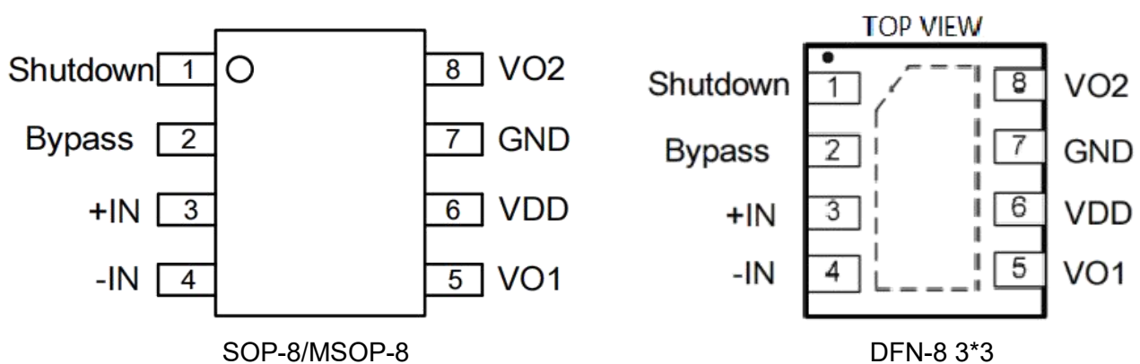
图 1. TS4871 的管脚定义图
