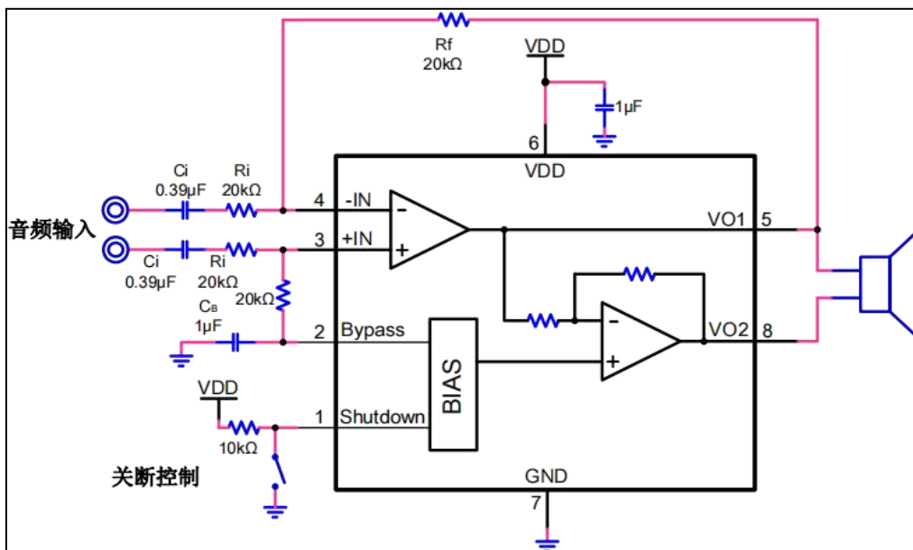
图 3. TS4871 差分输入模式电路图
