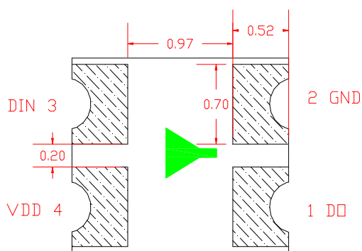
正面透视图
