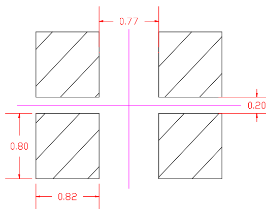
建议焊盘尺寸
