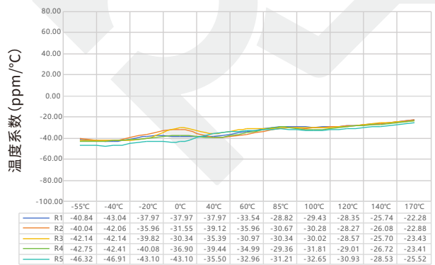
PEWF 系列 4026 规格 4.0mΩ 温度系数实测数据表
