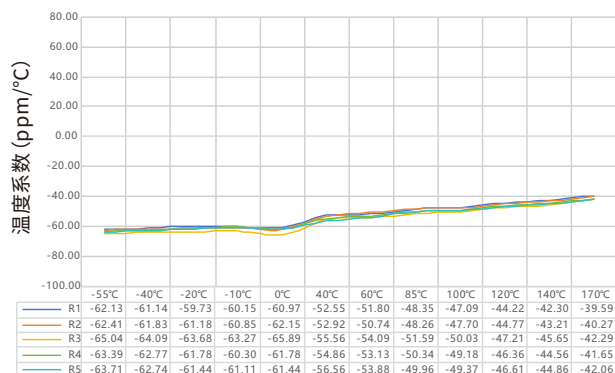
PEWF 系列 4026 规格 1.0mΩ 温度系数实测数据表
