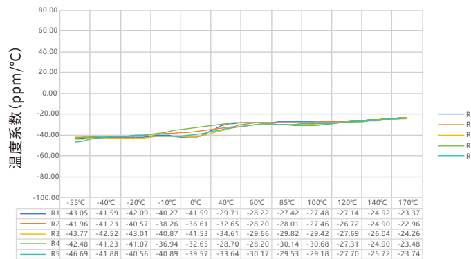
PEWF 系列 4026 规格 5.0mΩ 温度系数实测数据表
