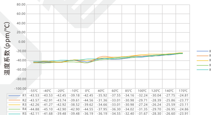
PEWF 系列 4026 规格 3.0mΩ 温度系数实测数据表
