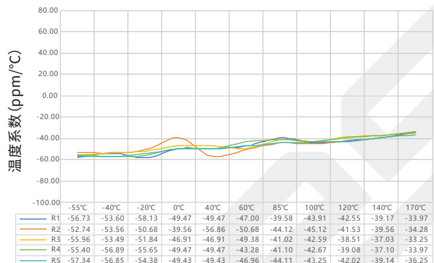
PEWF 系列 4026 规格 2.0mΩ 温度系数实测数据表
