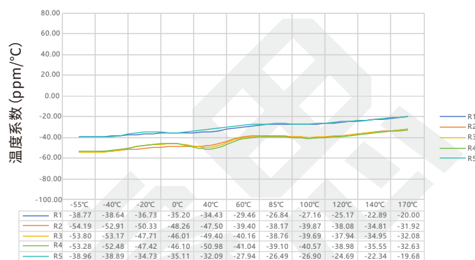
PEWF 系列 4026 规格 1.3mΩ 温度系数实测数据表
