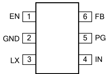
SOT23-6
