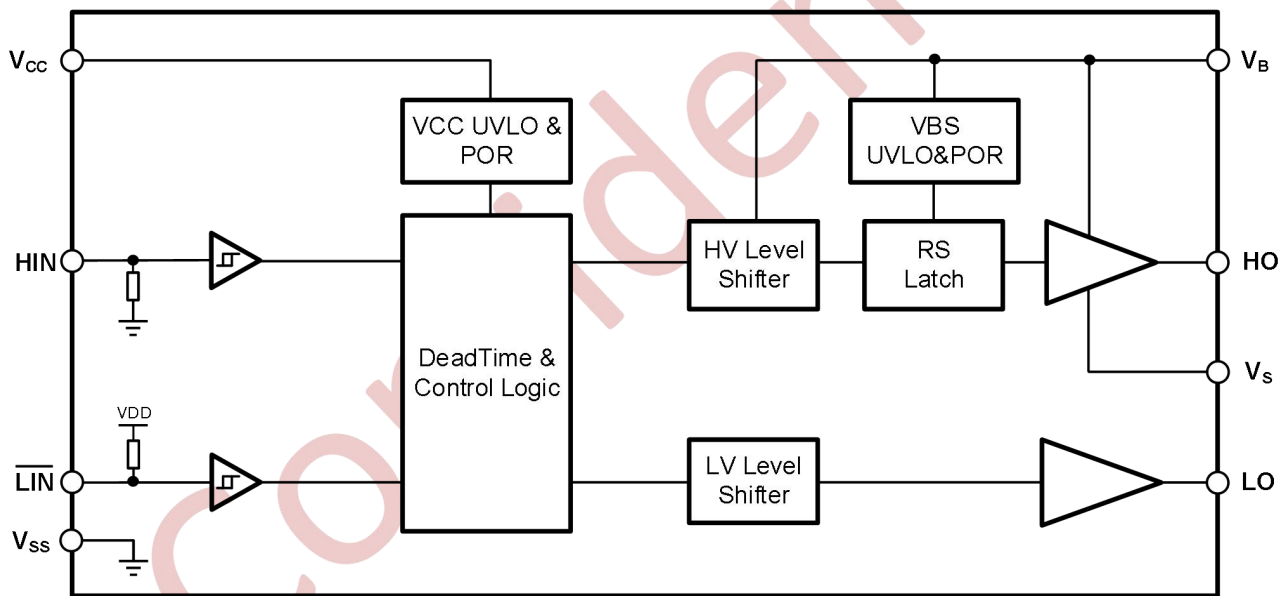
图 10-1 XJNG2103 功能框图
