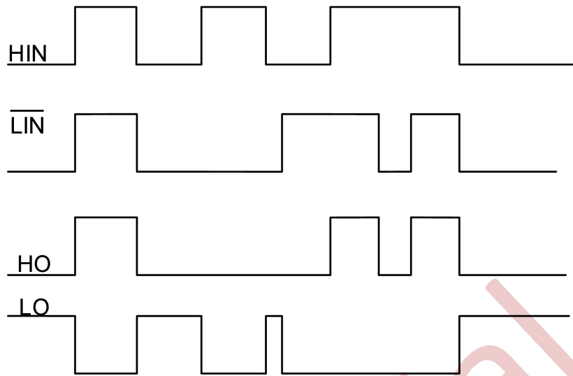
图 9-1 XJNG2103 输入输出时序波形
