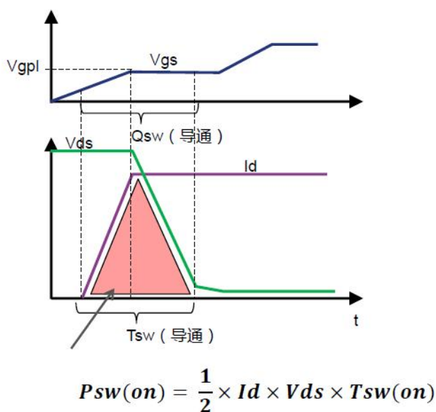
图 11-3 阻性负载条件下的 MOS 开关损耗
