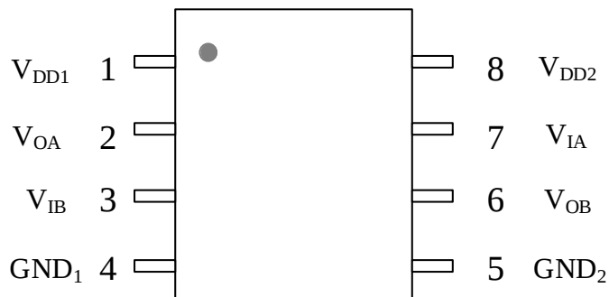
图 11-2 Gic1201 管脚分布
