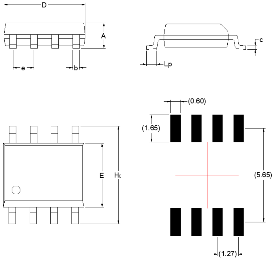
图 12-1 窄体 SOP8 封装外形图
