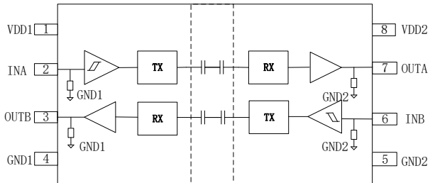
图4-6 Gic1211L原理框图
