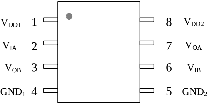
图 11-3 Gic1211 管脚分布
