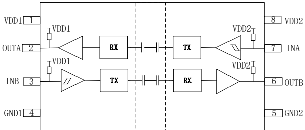
图4-3 Gic1201H原理框图
