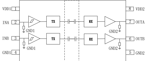
图4-2 Gic1200L原理框图
