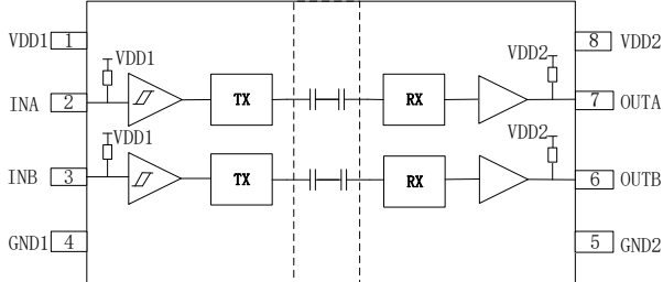
图4-1 Gic1200H原理框图
