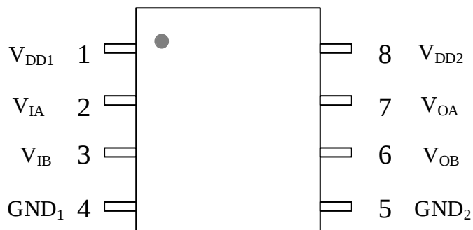
图 11-1 Gic1200 管脚分布
