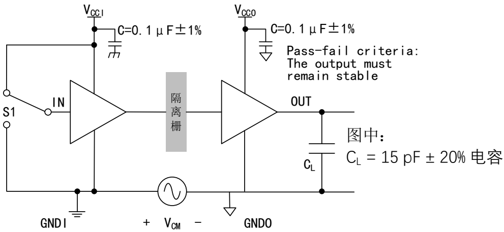
图 6-2 CMTI 测试电路
