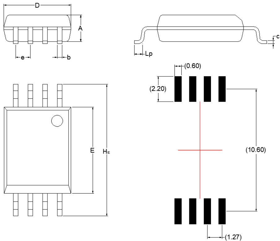
图 12-2 宽体 SOW8 封装外形图
