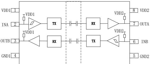
图4-5 Gic1211H原理框图
