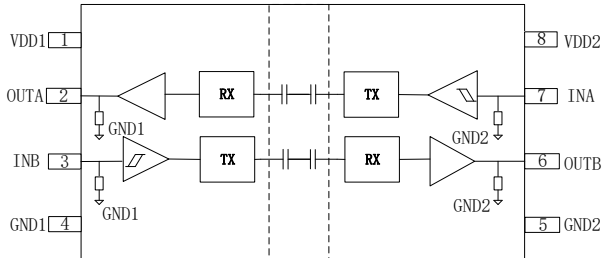
图4-4 Gic1201L原理框图
