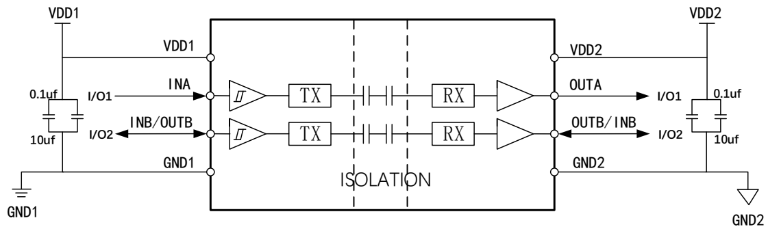
图 14-1 Gic120x 典型应用电路
