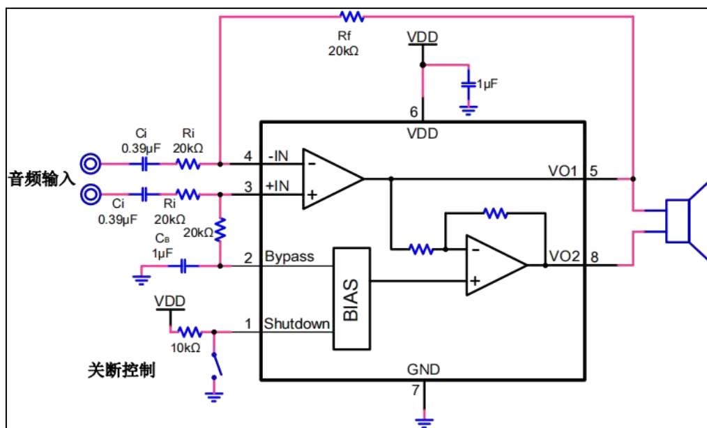
图 3. NCS2211 差分输入模式电路图
