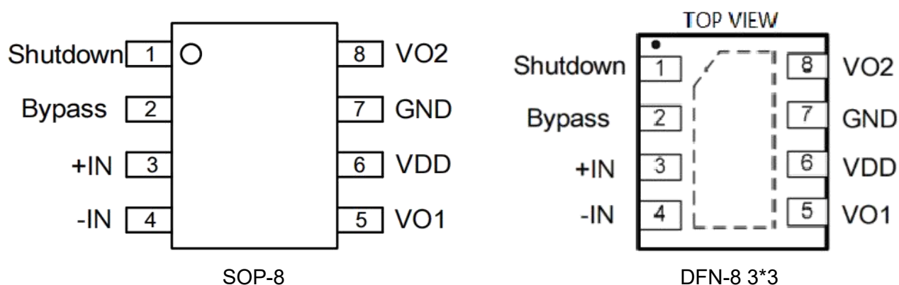
图 1. NCS2211 的管脚定义图
