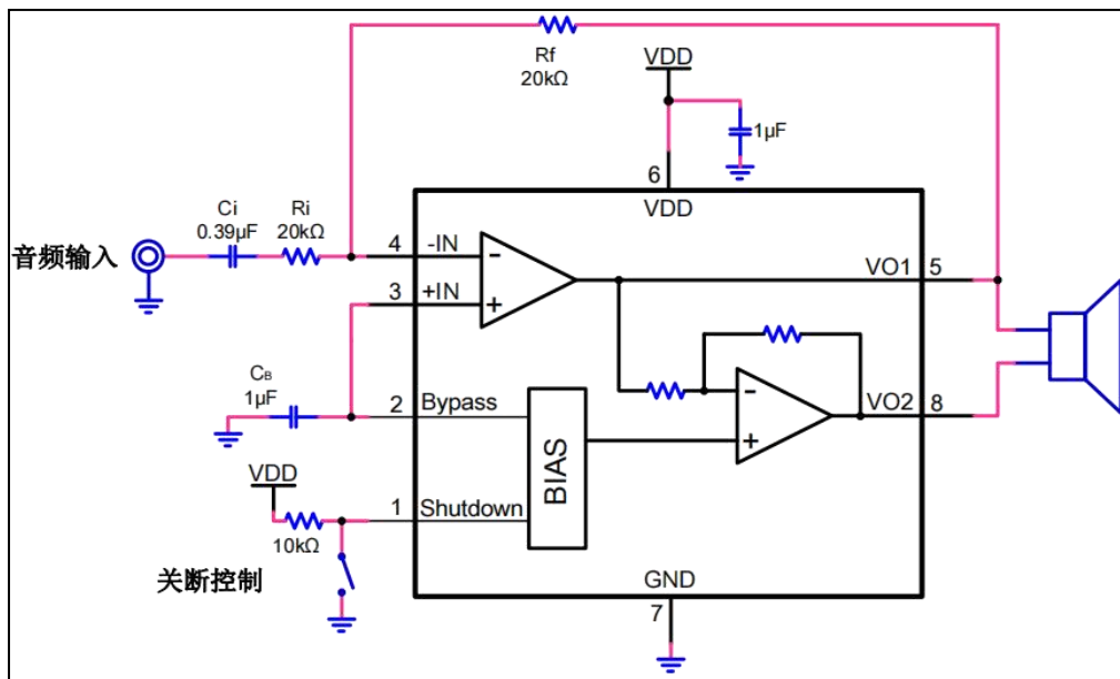
图 2. NCS2211 单端输入模式电路图
