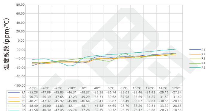
PEWF 系列 2726 规格 1.3mΩ 温度系数实测数据表
