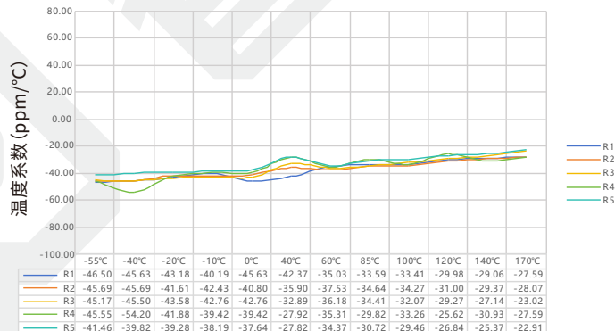
PEWF 系列 2726 规格 3.0mΩ 温度系数实测数据表
