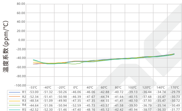
PEWF 系列 2726 规格 2.0mΩ 温度系数实测数据表
