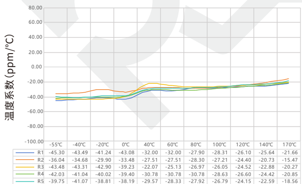
PEWF 系列 2726 规格 4.0mΩ 温度系数实测数据表
