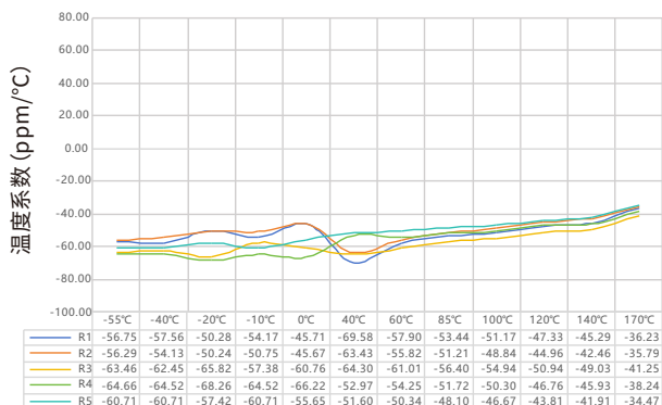
PEWF 系列 2726 规格 1.0mΩ 温度系数实测数据表
