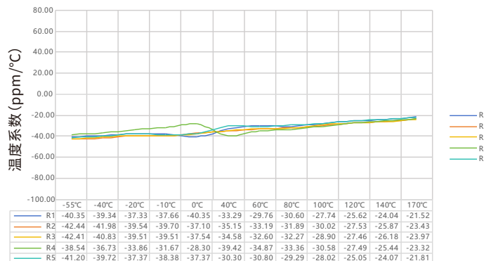
PEWF 系列 2726 规格 5.0mΩ 温度系数实测数据表
