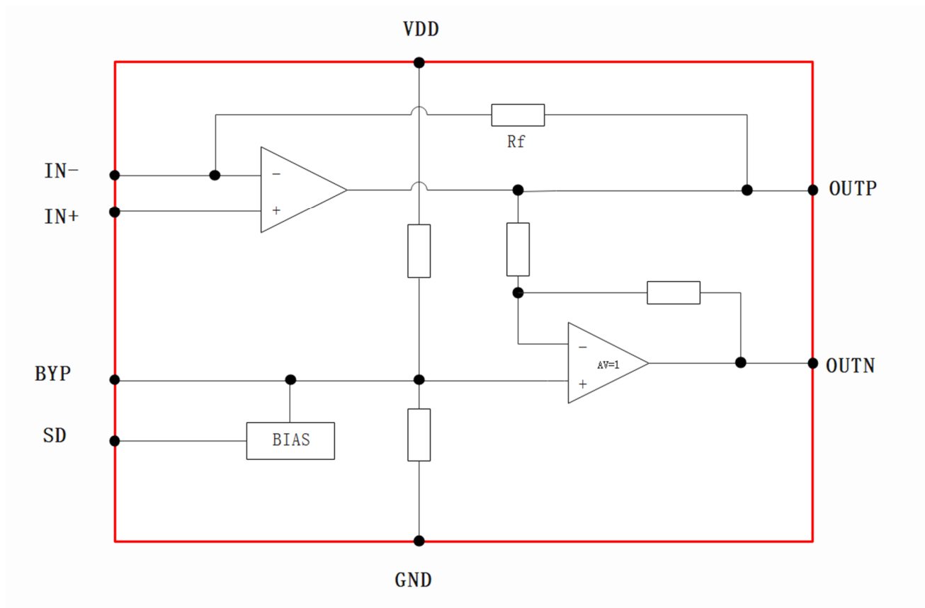
功能框图
