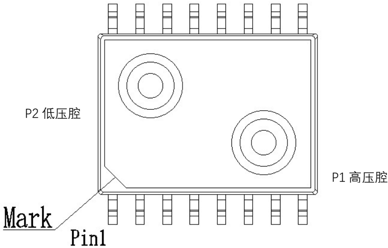
图 1. 引脚示意图
