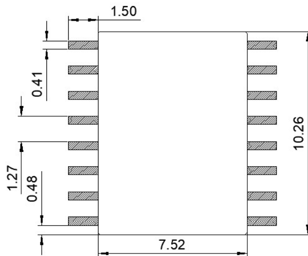
图7.推荐焊盘尺寸
