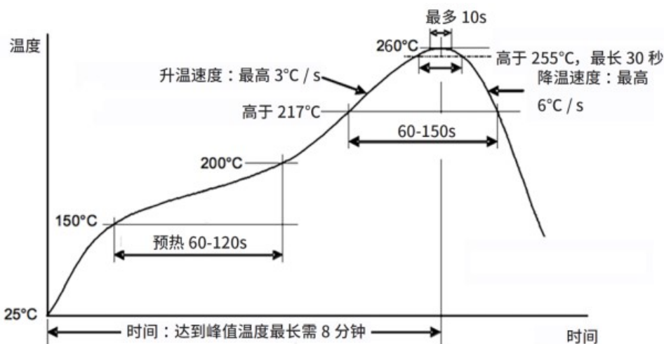
图 8.回流焊接
