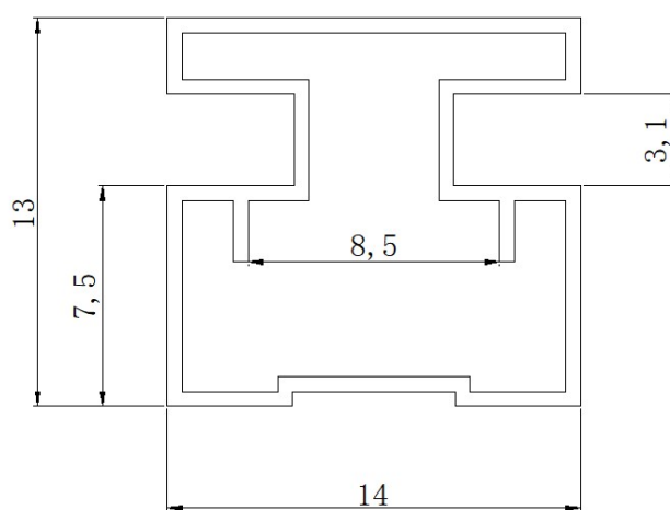
图 9.料管截面示意图
