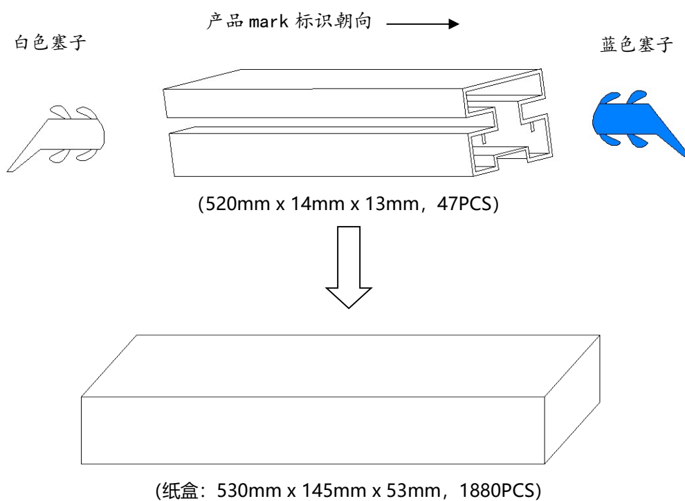
图 10.包装示意图
