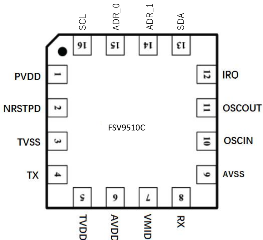
图 1 QFN16 3*3 封装管脚
