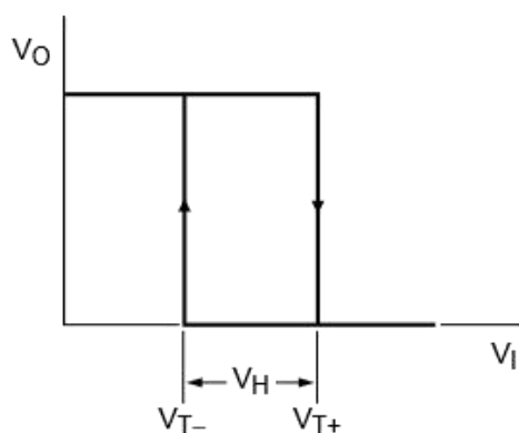
图 1、传输特性
