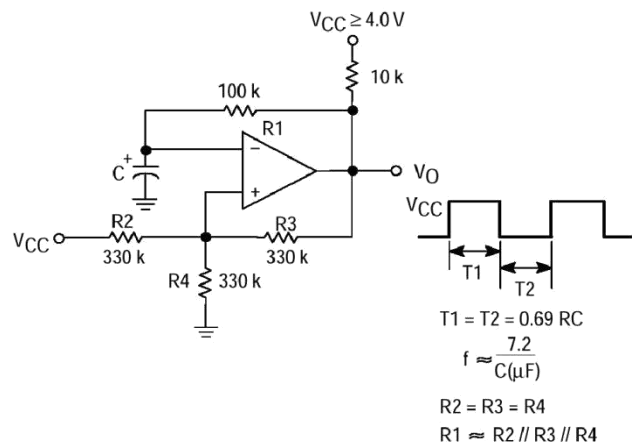
方波振荡器
