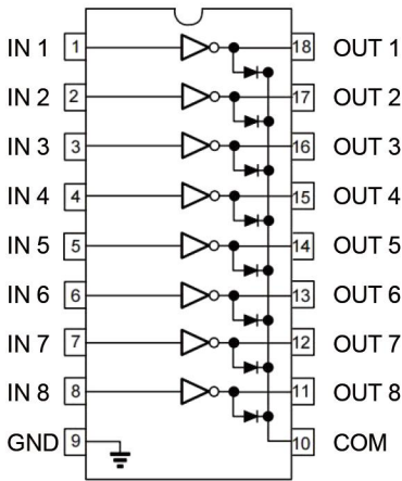
ULN2803A 管脚说明表
