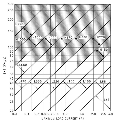
LM2576HV-ADJ
